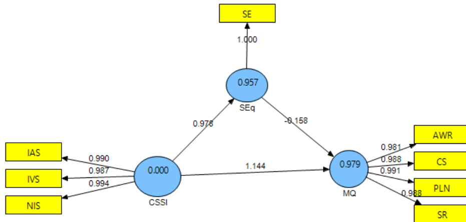
شکل (۲) مدل ساختاری تحقیق در حالت استاندارد
